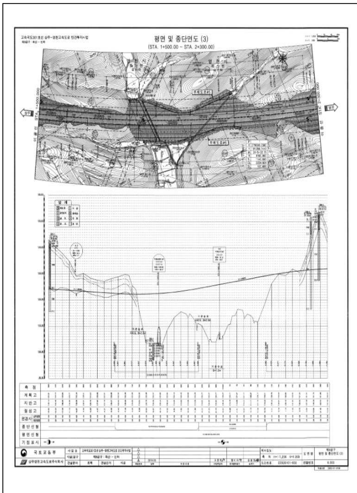
【그림 62.3】 평면도
